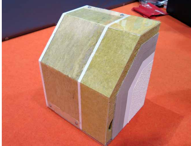
Provedení a celková skladba obvodové stěny z konstrukčních panelů GOOPAN PLUS
