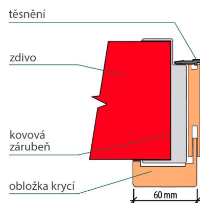
Částečný obklad ocelové zárubně
