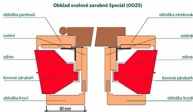
Obklad ocelové zárubně Speciál (OOZS)
