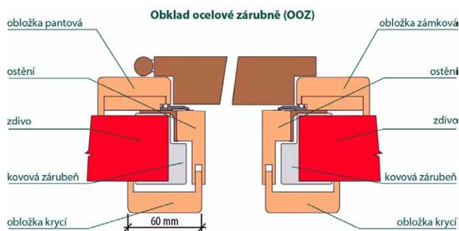
Obklad ocelové zárubně (OOZ)
