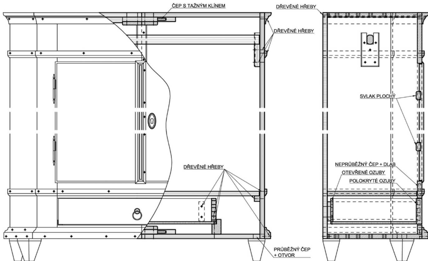
Konstrukční výkres dvoudveřové skříně (Nb 145)
