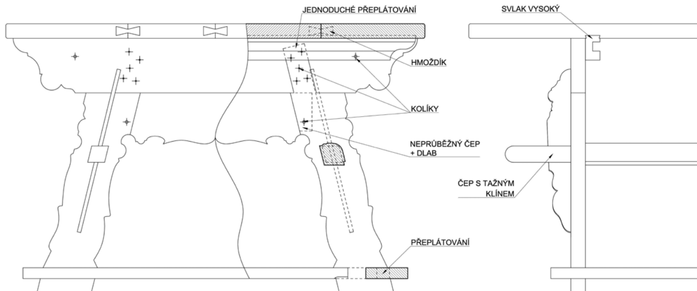
Konstrukční výkres jídelního stolu
