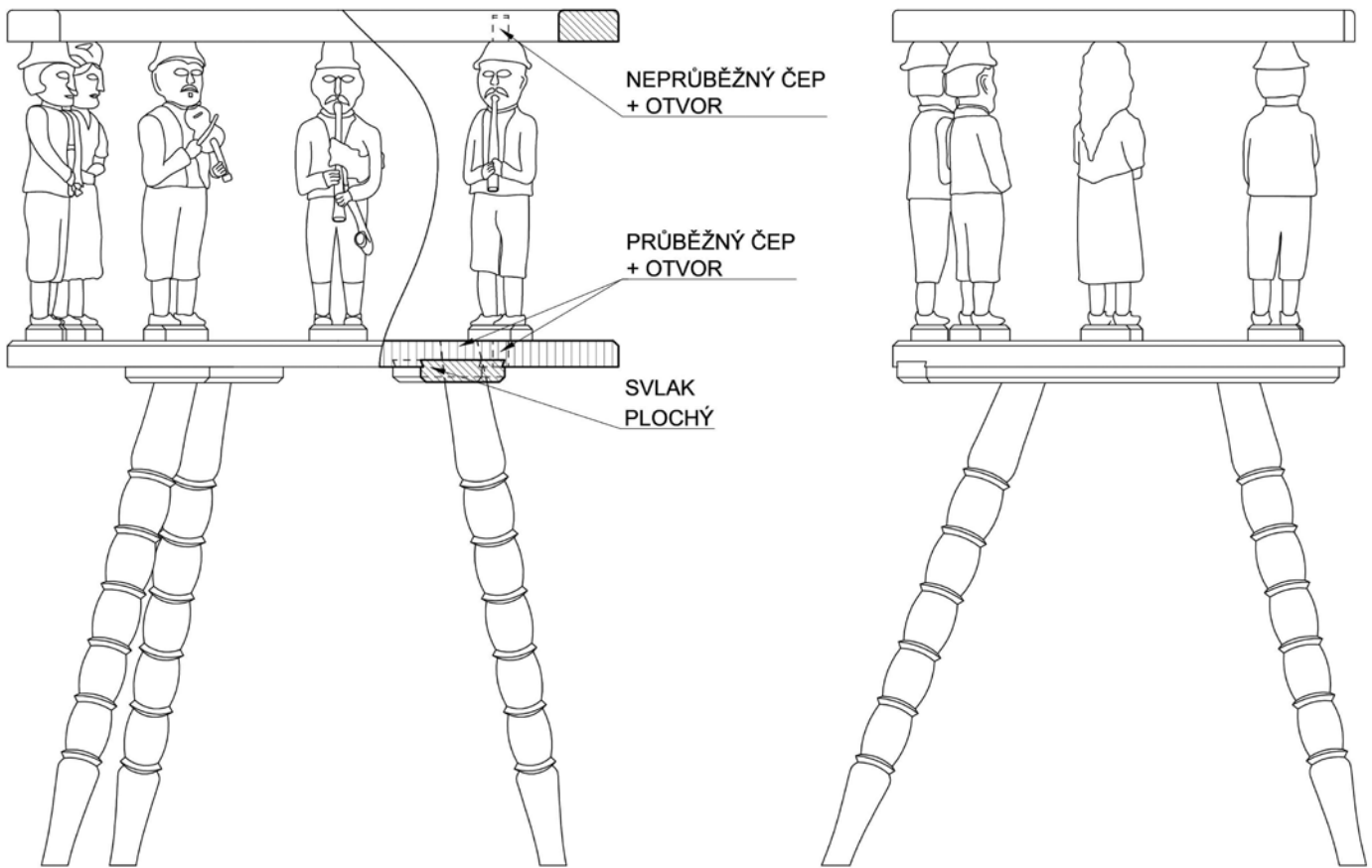
Konstrukční výkres polokruhového křesla (Nb 24)
