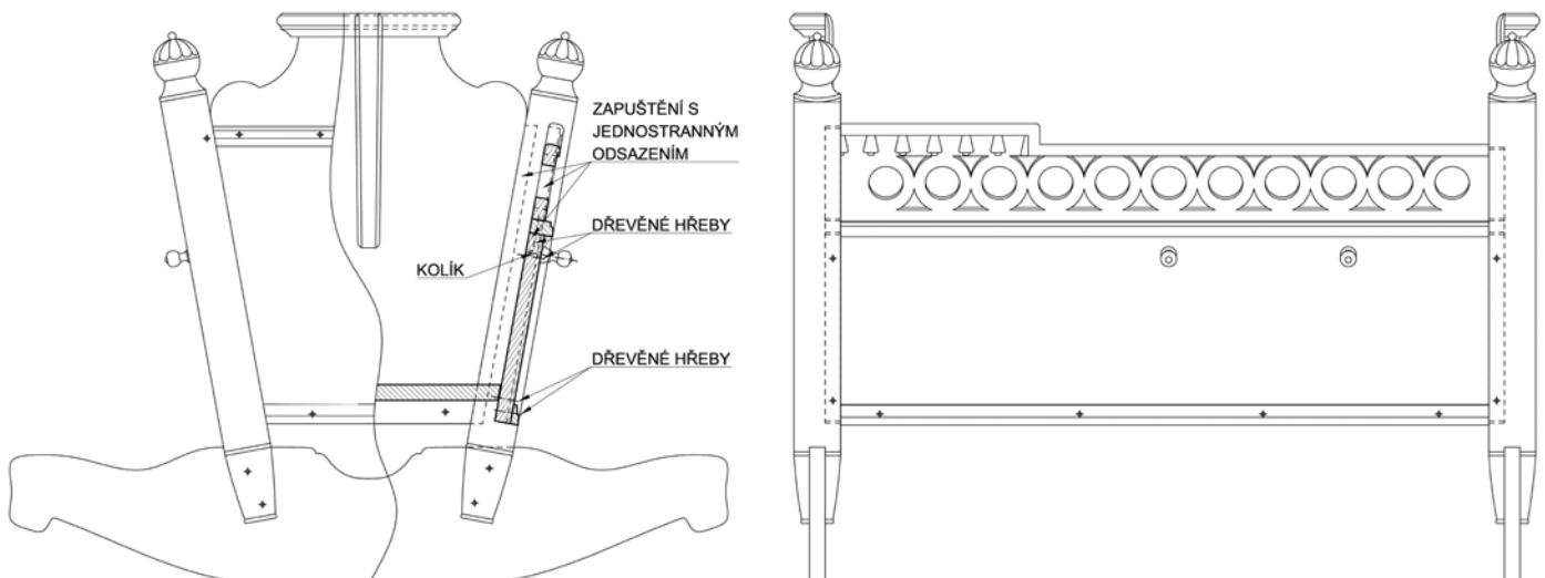
Konstrukční výkres kolébky
